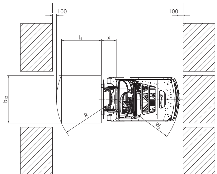
Bovenaanzicht 3 wielen
