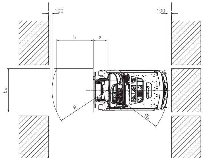
Bovenaanzicht 4 wielen
