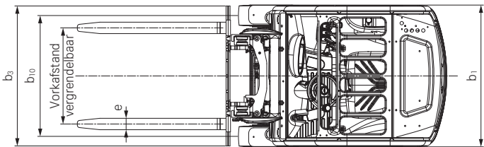
RXE bovenaanzicht
