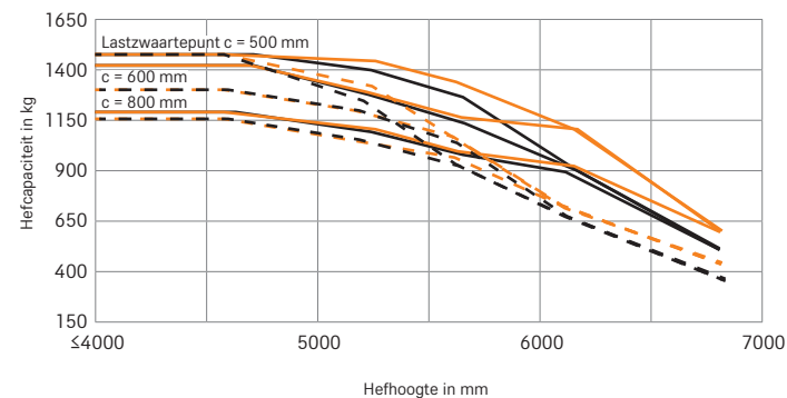
RXE 16C Drievoudige mast – enkele superelastische banden 180/70-8, Voertuigbreedte 990 mm + 1028 mm
