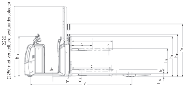
Zijaanzicht OPX-L 20
