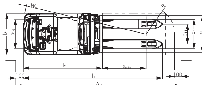
Bovenaanzicht OPX-D 20
