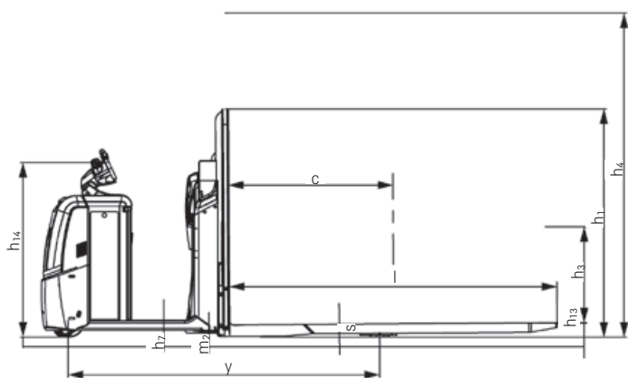
Zijaanzicht OPX-L 16
