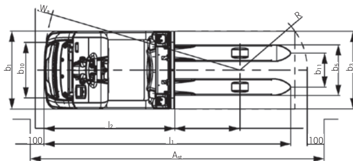
Bovenaanzicht OPX-L 12
