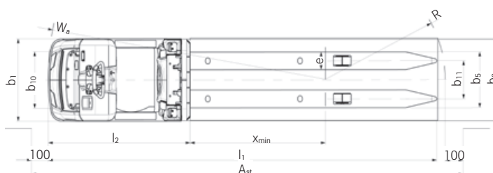
Bovenaanzicht OPX-L 20 S
