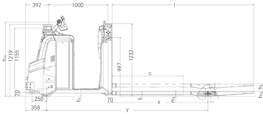
Zijaanzicht OPX 20 iGo neo
