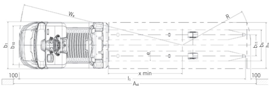
Bovenaanzicht OPX-L 20 S iGo neo
