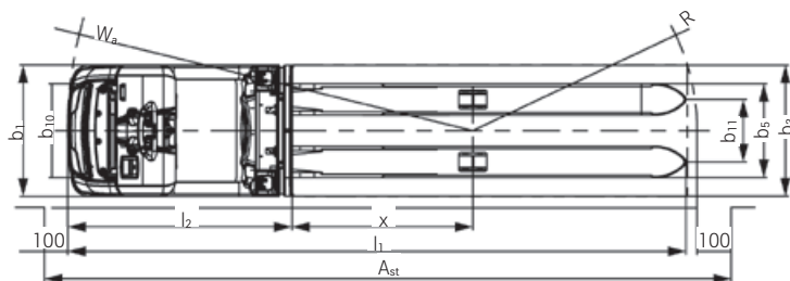
Bovenaanzicht OPX-L 16
