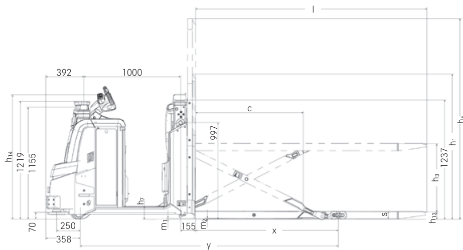
Zijaanzicht OPX-L 20 S iGo neo
