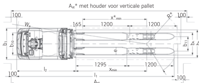
Bovenaanzicht OPX-L 20
