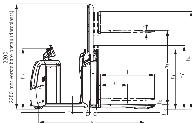
Zijaanzicht OPX-D 20
