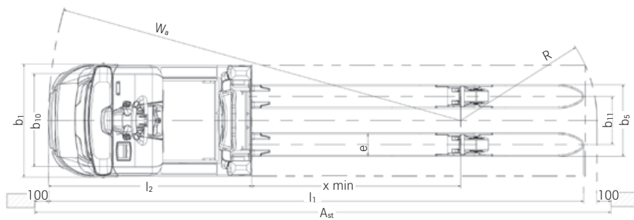
Bovenaanzicht OPX 20 iGo neo
