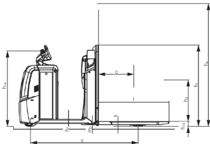
Zijaanzicht OPX-L 12
