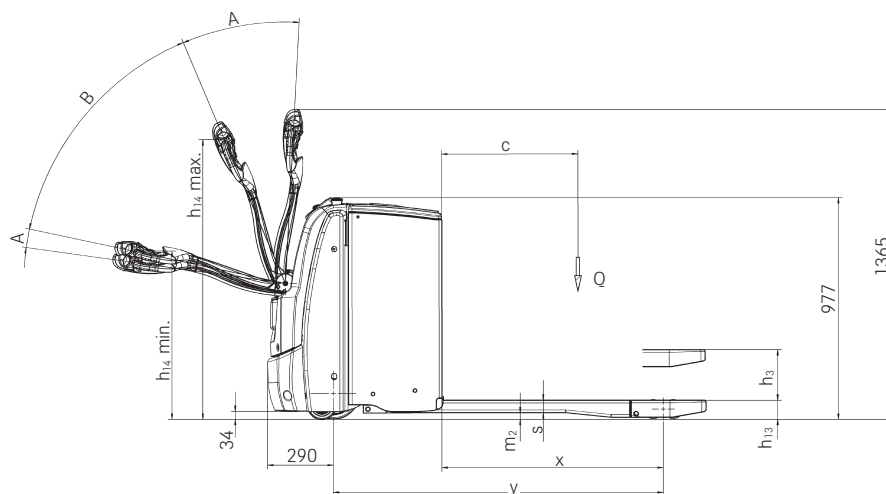
Zijaanzicht EXH 25/30
