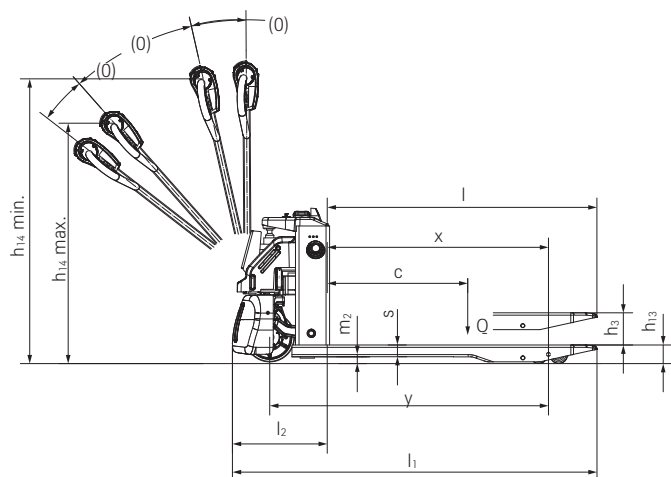
ECH 12C/15C zijaanzicht
