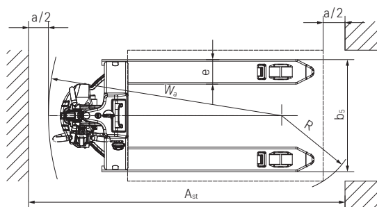
ECH 12C/15C bovenaanzicht
