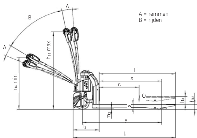
ECH 12 zijaanzicht
