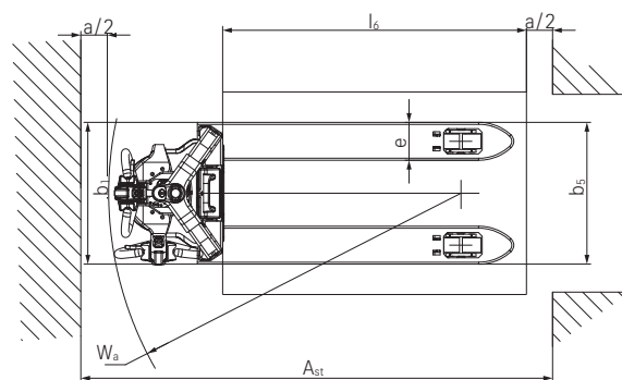
ECH 12 bovenaanzicht
