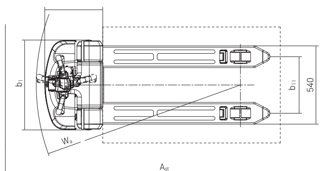
ECH 15 bovenaanzicht
